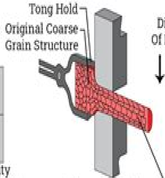
Open Die
