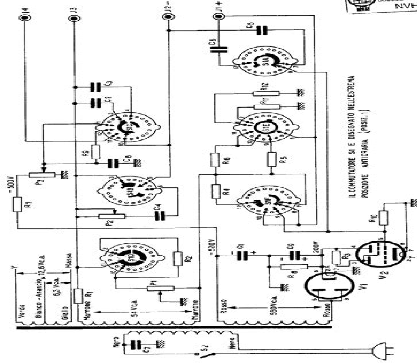
Fig. 1 - Schema elettrico del comparatore a Ponte Mod. 950 B.
